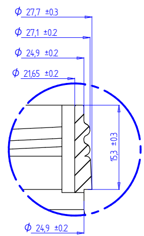
DETAIL A 2:1 PILFERPROOF 28 STD
