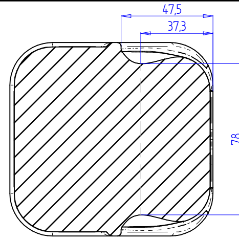
CORTE A-A
