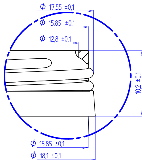
PILFERPROOF 18 STD DETAIL NECK 3:1
