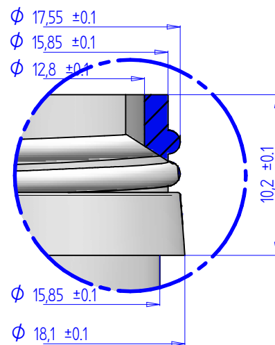
PILFERPROOF 18 STD DETAIL NECK A 3:1
